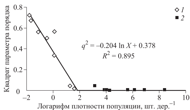
Рис. 2. Связь между квадратом доли неповрежденных деревьев q^2 и логарифмом плотности X популяций сибирского шелкопряда в очагах массового размножения в 1953–1969 гг. (Кондаков, 1974).
