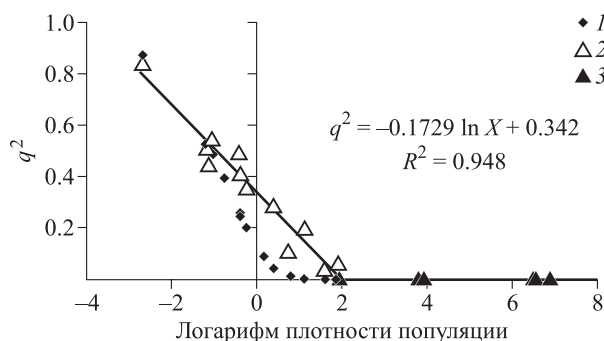
Рис. 4. Связь квадрата доли незаселенных деревьев на пробных площадях и логарифма плотности популяции в очагах массового размножения сибирского шелкопряда на территории Восточной Сибири (Болдаруев, 1969).
