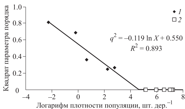
Рис. 3. Связь между квадратом доли неповрежденных деревьев q^2 и логарифмом плотности X популяций сибирского шелкопряда в очагах массового размножения на территории Красноярского края в 2017 г.
