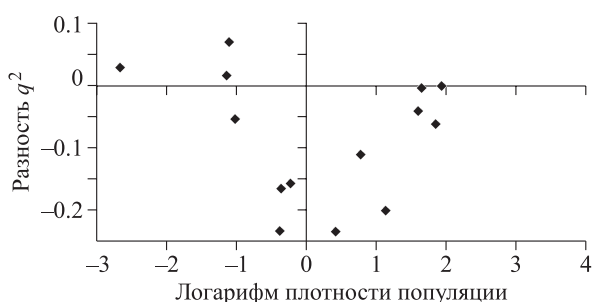
Рис. 5. Разность между пуассоновской моделью распределения гусениц по деревьям и моделью фазового перехода второго рода.
